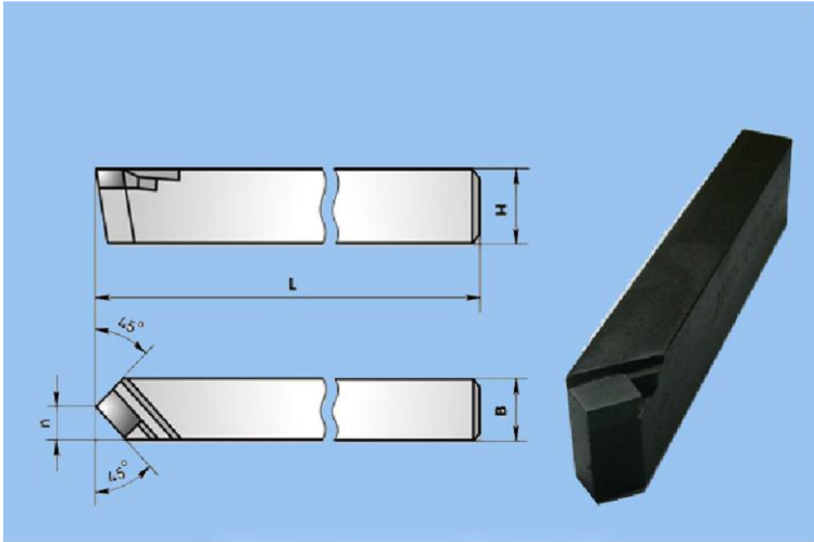
Նկ. 3.17. Ուղիղ գլխիկով անցումային կտրիչ
