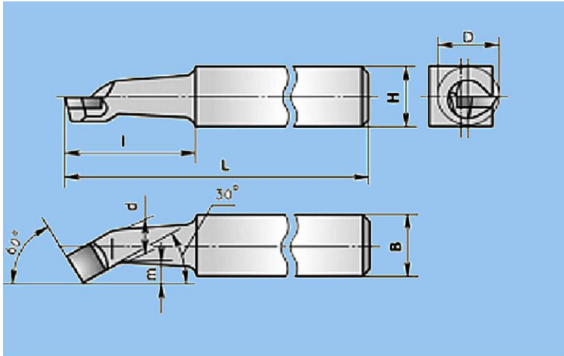
Նկ. 3.21. Անցողիկ անցքի ներտաշ կտրիչ
