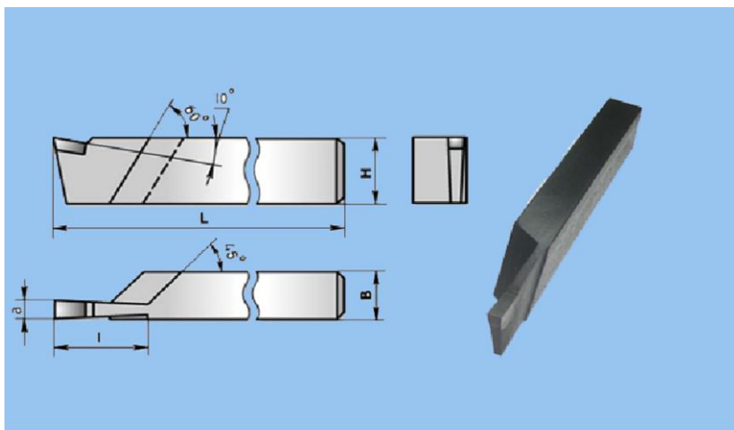
Նկ. 3.24. Խառատային հատիչ կտրիչ
