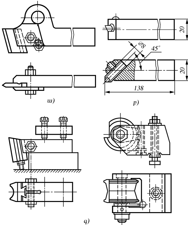
Նկ. 3.4. Խառատային հաստոցի բռնիչ ա) պարուրակահան կտրիչի համար, բ) ներտաշ կտրիչի համար, գ) ձևավոր կտրիչների համար
