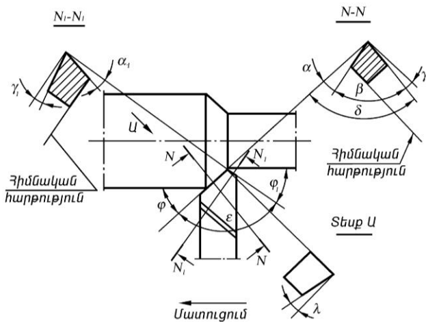
Նկ. 3.15. Կտրիչի երկրաչափական պարամետրերը
