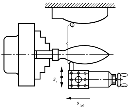
Նկ. 3.9. Երկայնակի մատուցման եղանակով ձևավոր մակերևույթի մշակման սխեման
