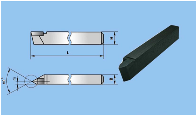
Նկ. 3.22. Արտաքին պարուրակի մշակման կտրիչ
