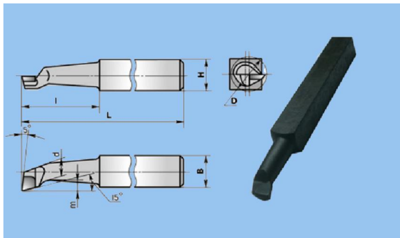
Նկ. 3.20. Անցումային ներտաշ կտրիչ
