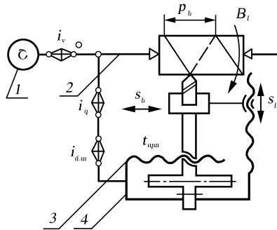
Նկ. 3.1.1. Խառատա-պտուտակահան հաստոցի կառուցվածքային սխեման
