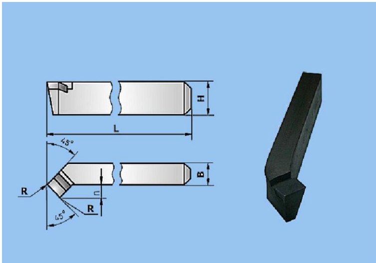
Նկ. 3.18. Թեքված գլխիկով անցումային կտրիչ
