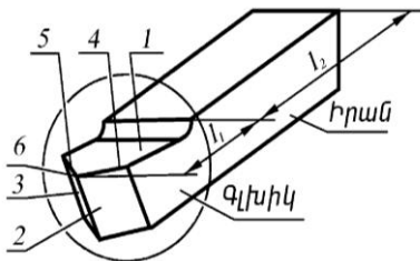
Նկ. 3.12. Նորմալ կտրիչի տարրերը
