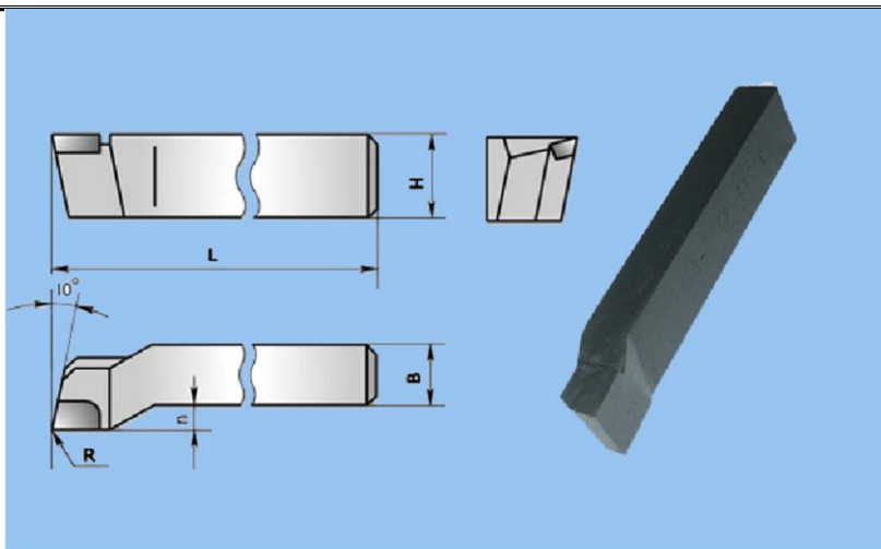
Նկ. 3.19. Դիմադիր անցումային կտրիչ
