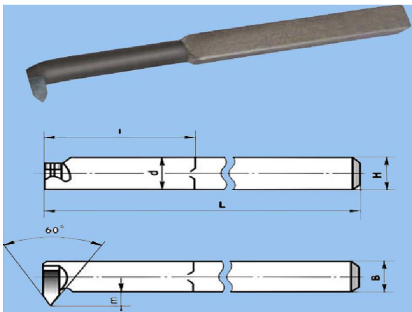
Նկ. 3.23. Ներքին պարուրակի մշակման կտրիչ
